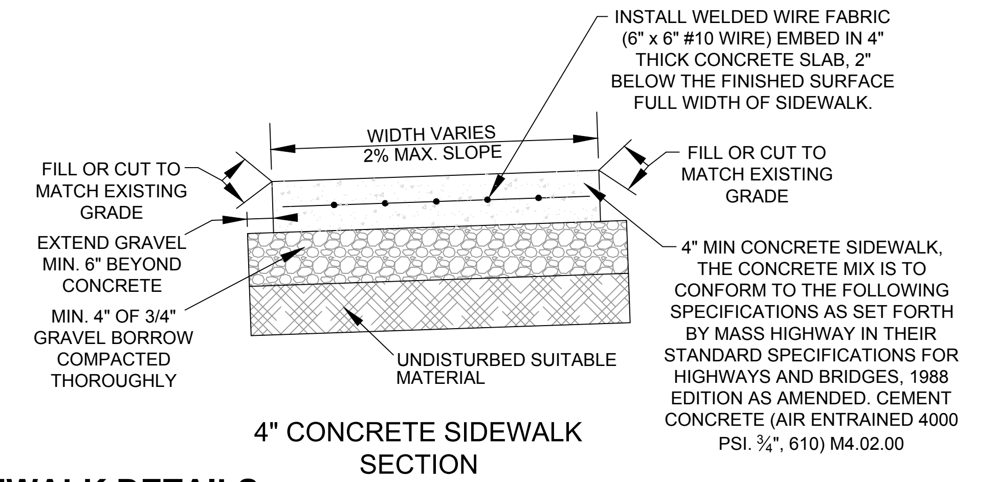
SIDEWALK DETAILS (SCALE: N.T.S.)
